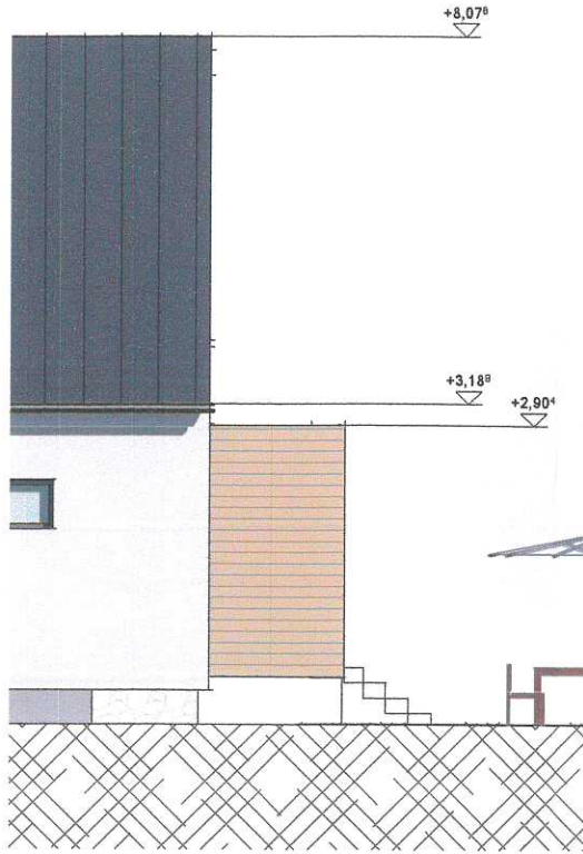
Ansicht Ost
