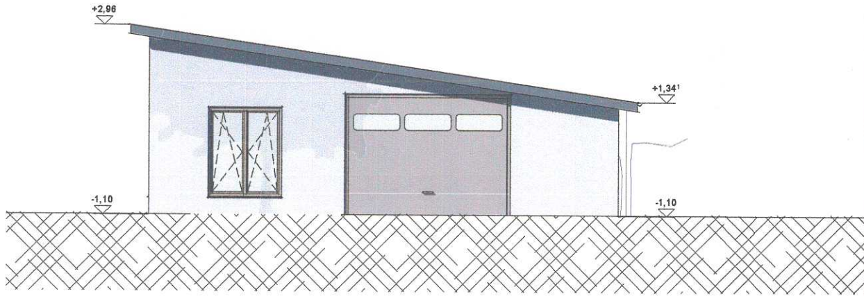
Ansicht Süd
