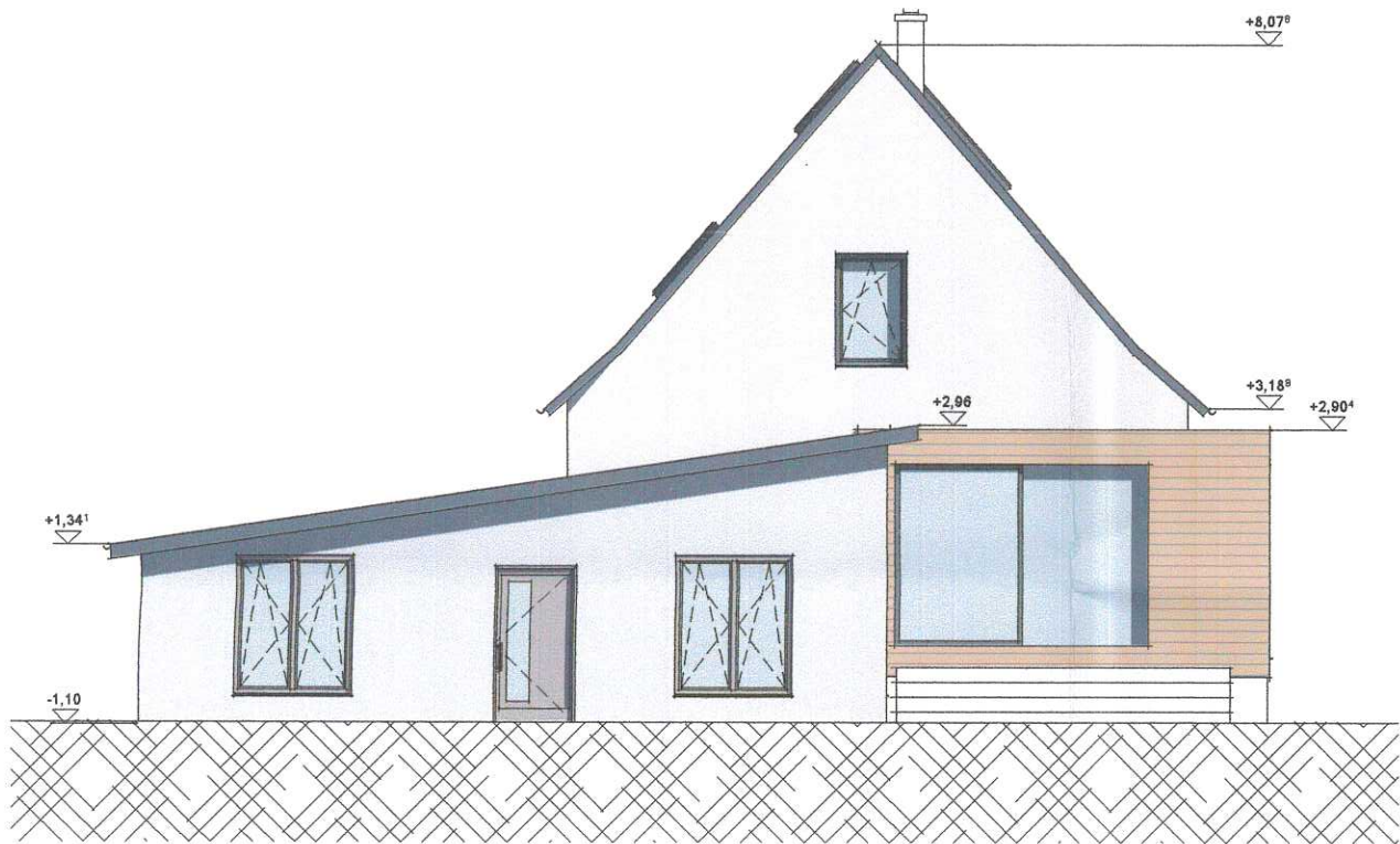
Ansicht Nord
