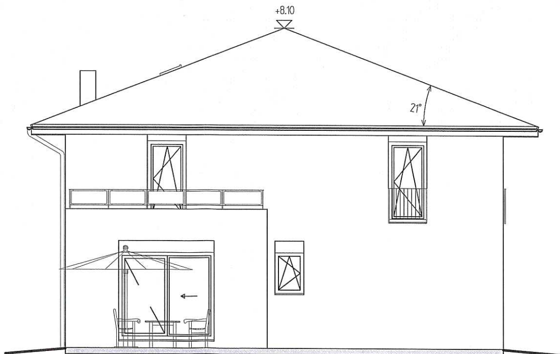
Ansicht Ost
