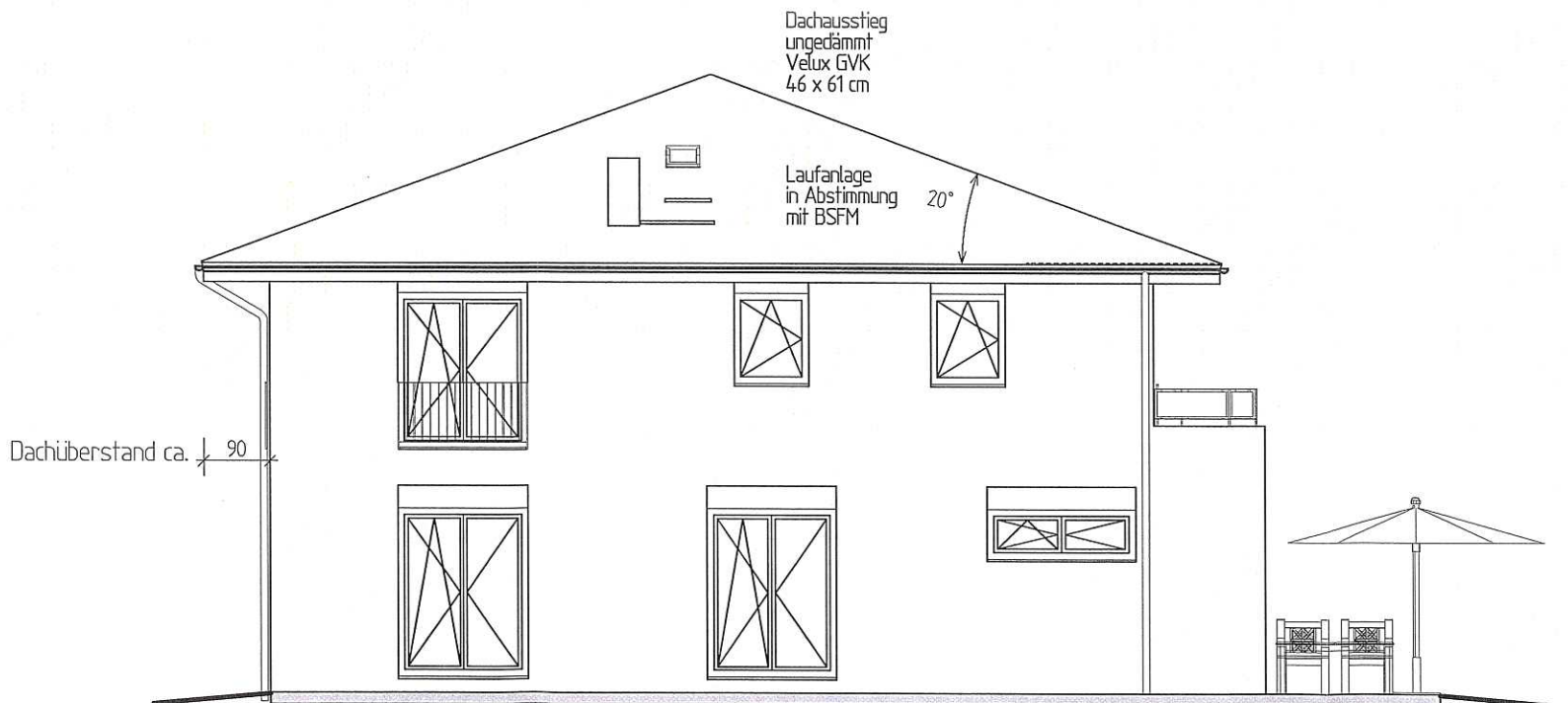
Ansicht Nord
