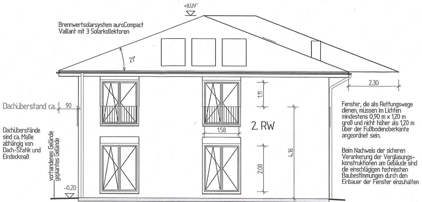
Ansicht West
