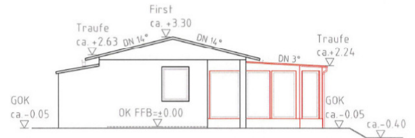
Nordwestfassade
