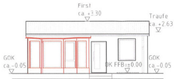
Südwestfassade
