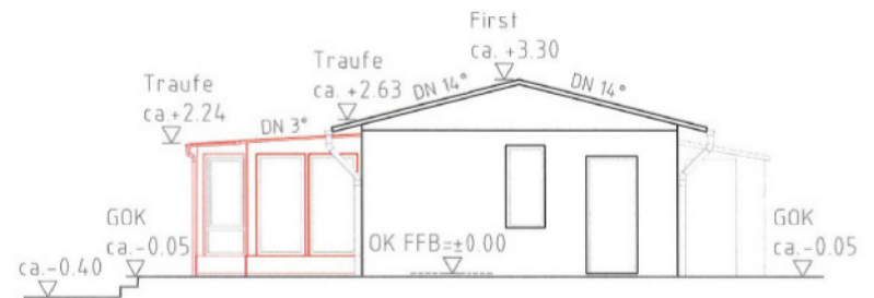
Südostfassade
