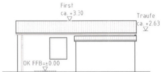
Nordostfassade
