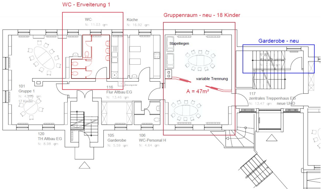
Grundriss EG
